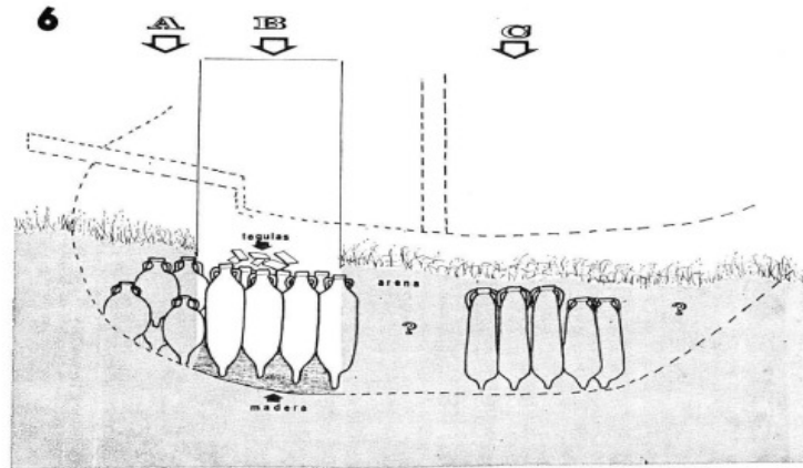
FIGURA 6 Hipótesis de reconstrucción del cargamento del barco CABRERA-1:
